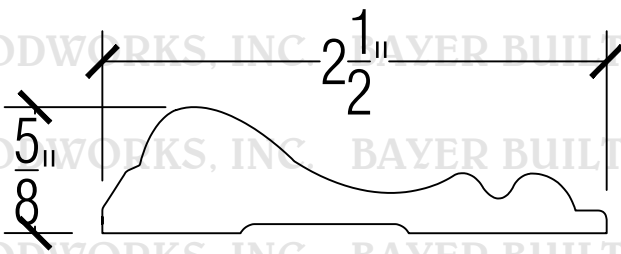
720A PANEL MOULD
